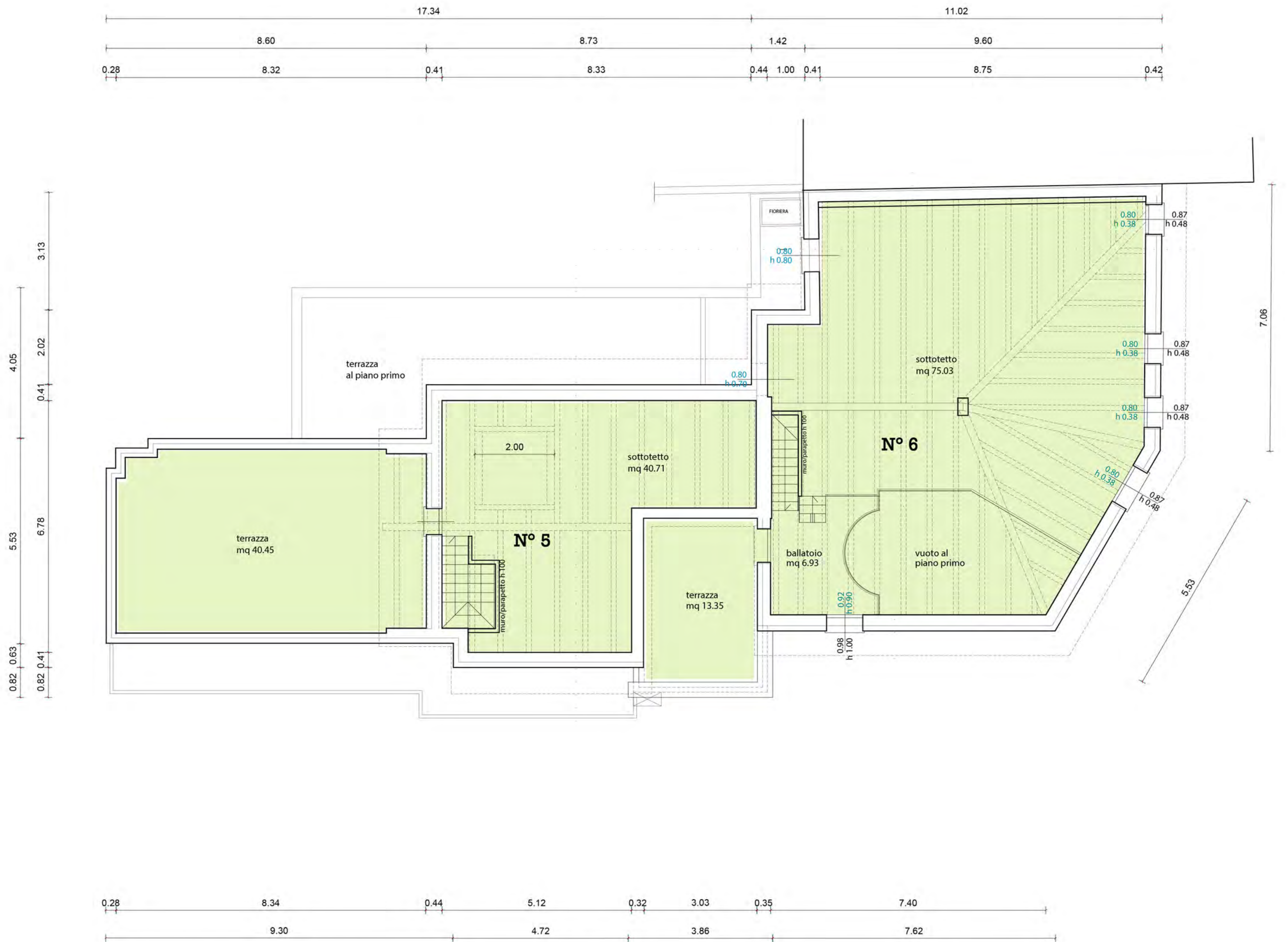
PIANTA PIANO SOTTOTETTO
