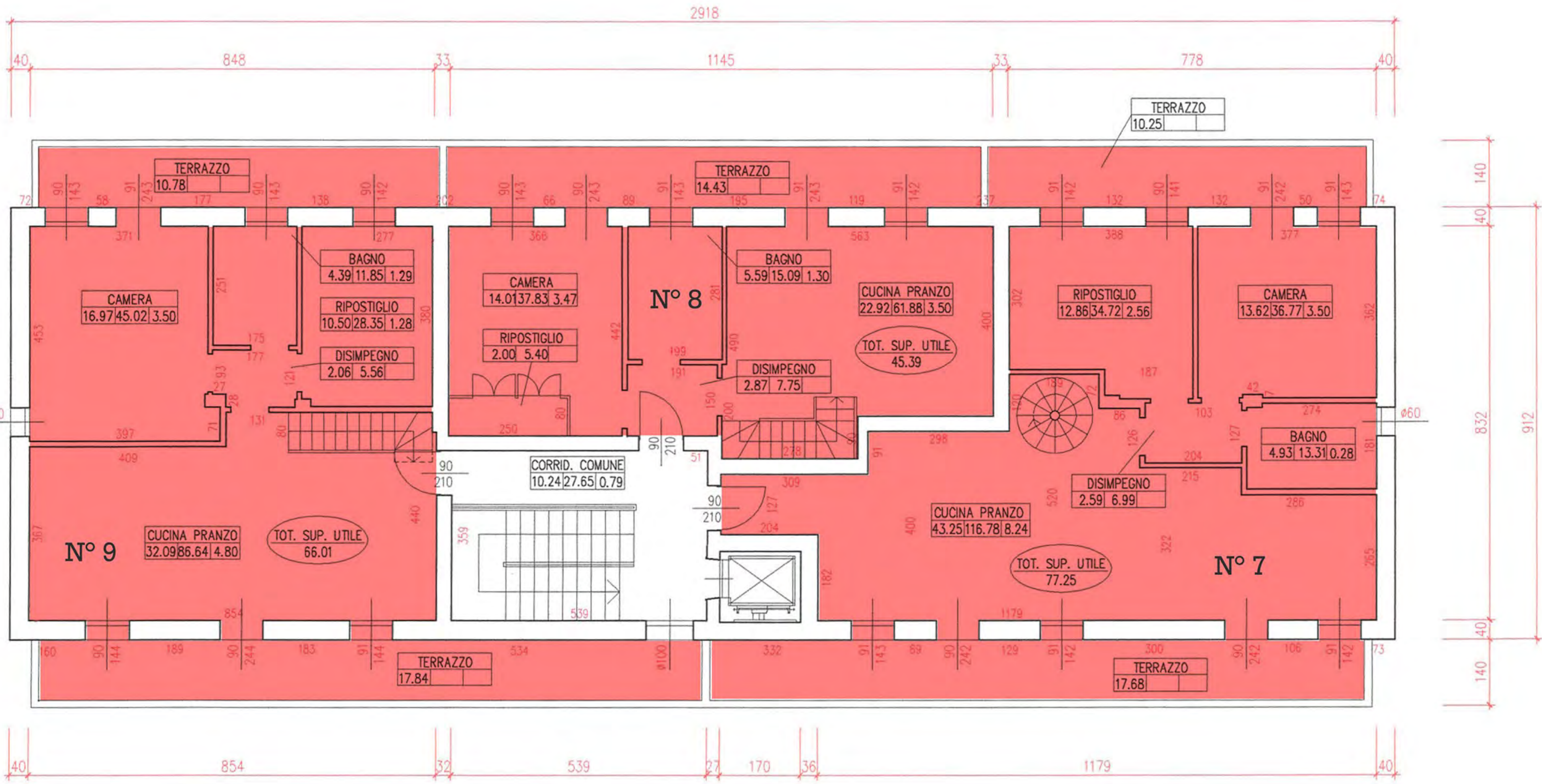
TERZO PIANO sc. 1:100
